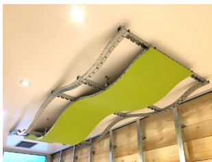
Bild 3: Välvda undertak
